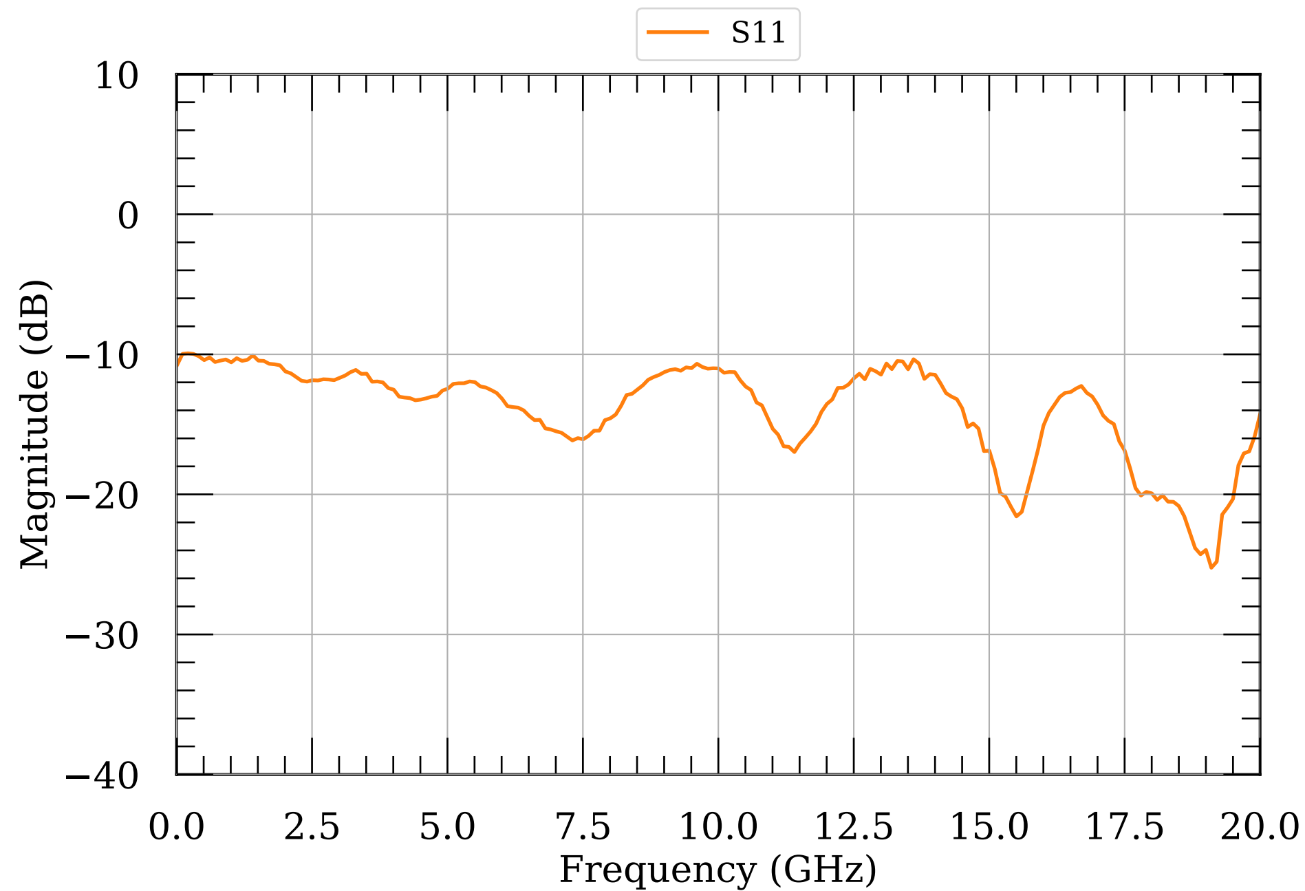
LNA S-params module060
